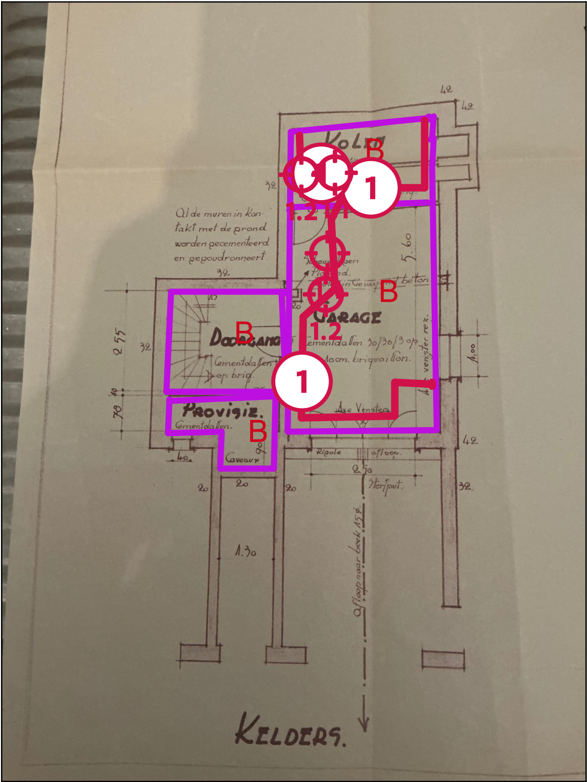
Legende van plan 1.2: Kelderverdieping
