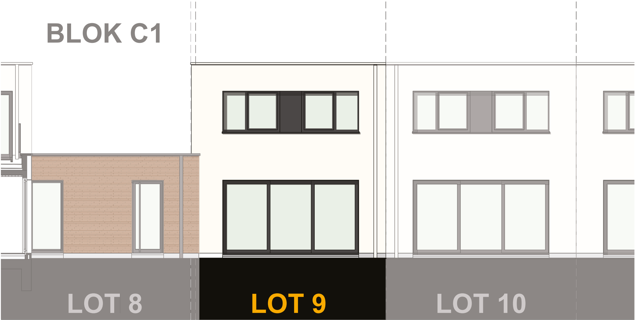
ACHTERGEVEL
