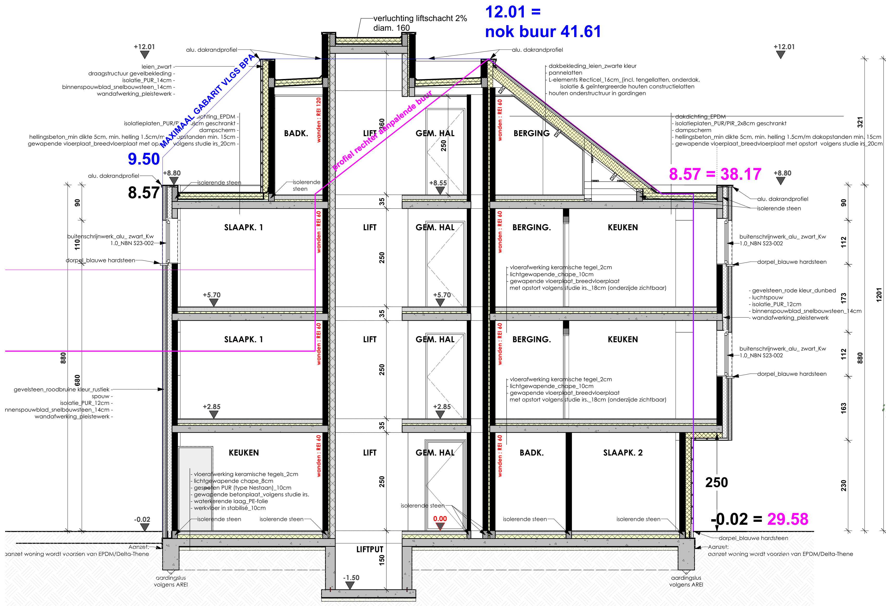
DOORSNEDE 1-2 schaal: 1/50
