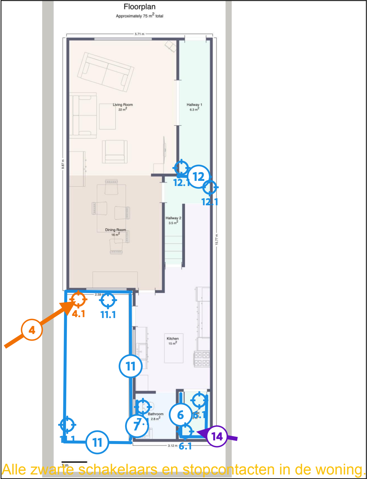
Legende van plan 1.3: Plan gelijkvloers
