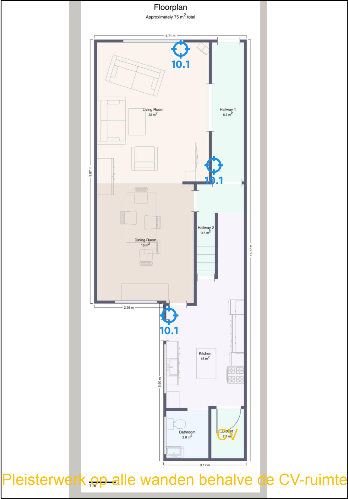
Legende van plan 1.2: Plan pleisterwerk gelijkvloers
