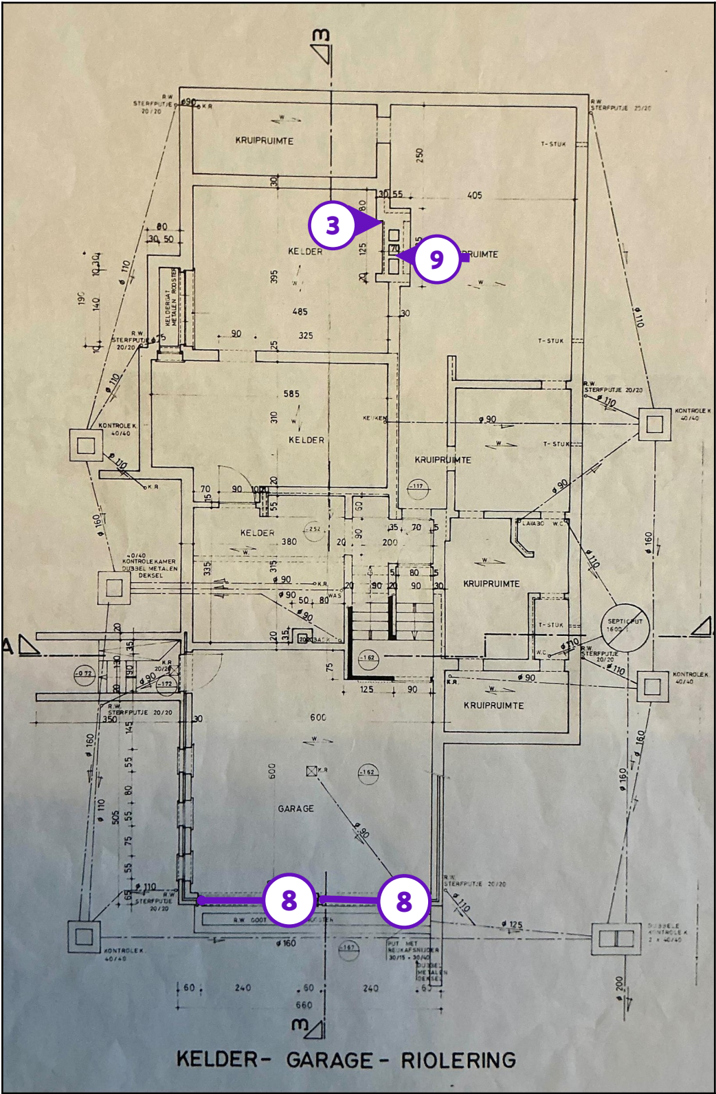
Legende van plan 1.1: Kelder plan
