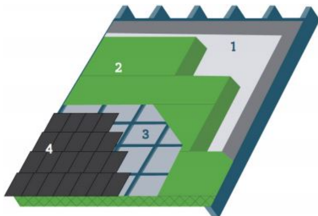
1. Dampscherm | 2. Isolatatie | 3. Onderdak | 4. Dakbekleding
